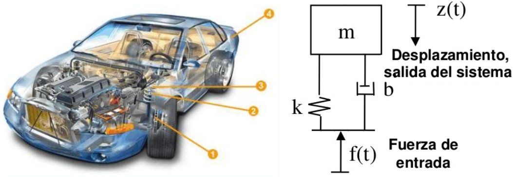
Figura 31. Modelo del sistema de suspensión
