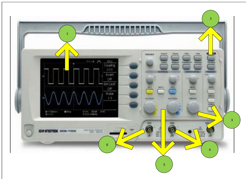
Figura 17. Osciloscopio digital.
