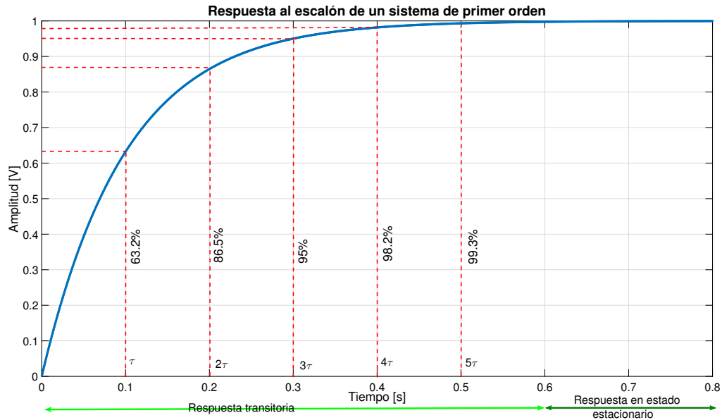
Figura 33. Respuesta de un sistema de 1 er orden
